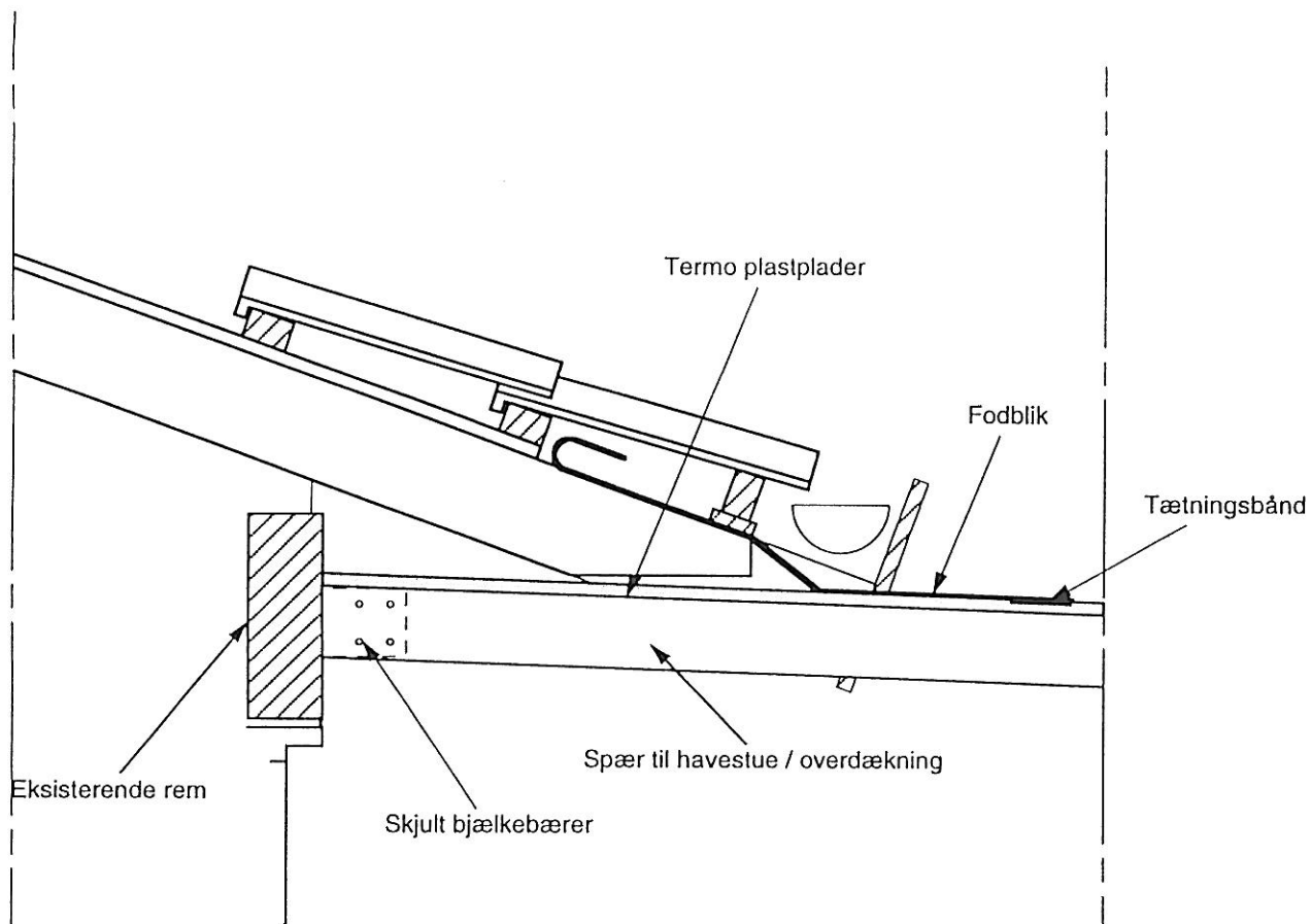
Spærtilslutning til eksisterende rem.
